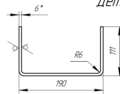
Дет. поз. 5
