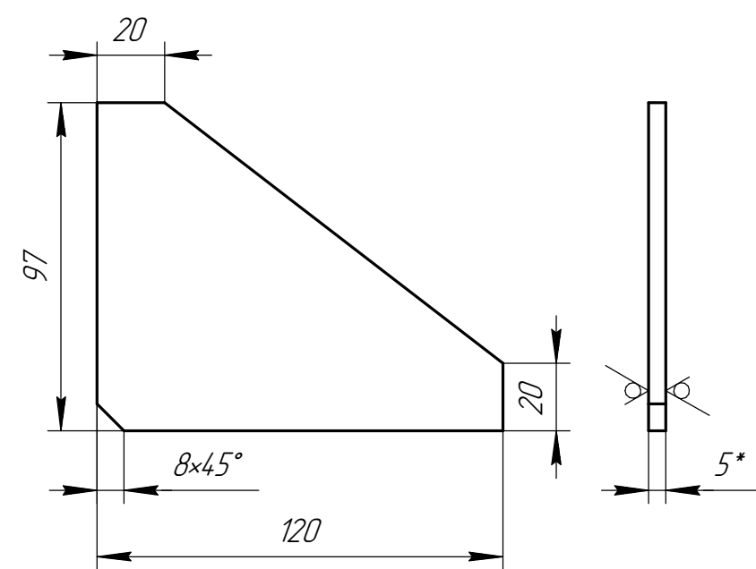
Дет. поз. 6 (1:2)
