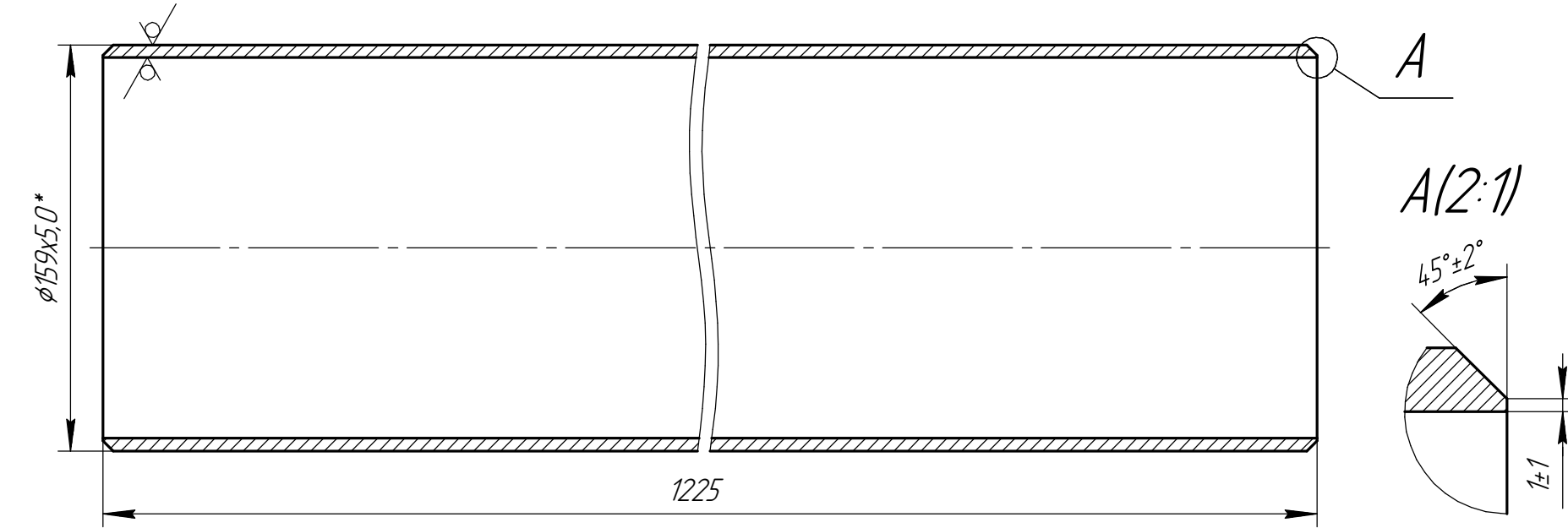
Дет. поз. 1 (1:2,5)
