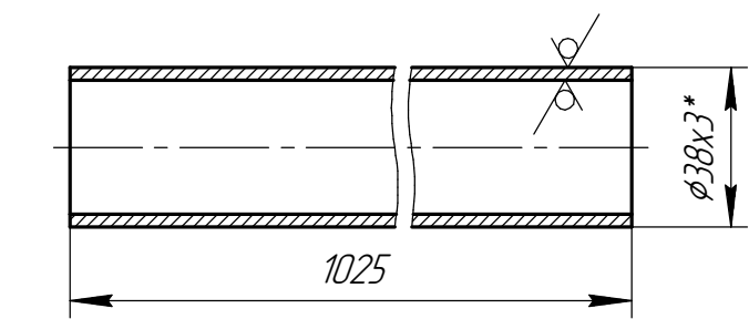
Дет. поз. 10 (1:2)
