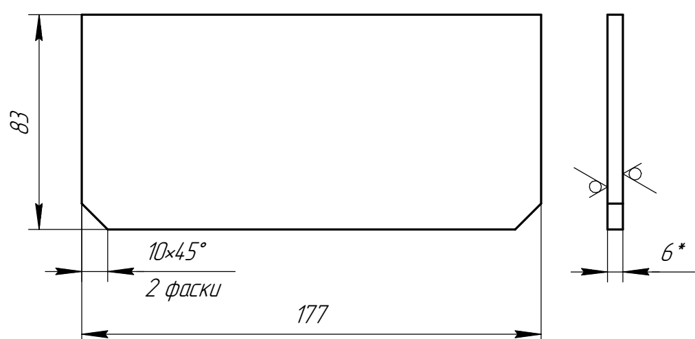
Дет. поз. 5 (1:2)
