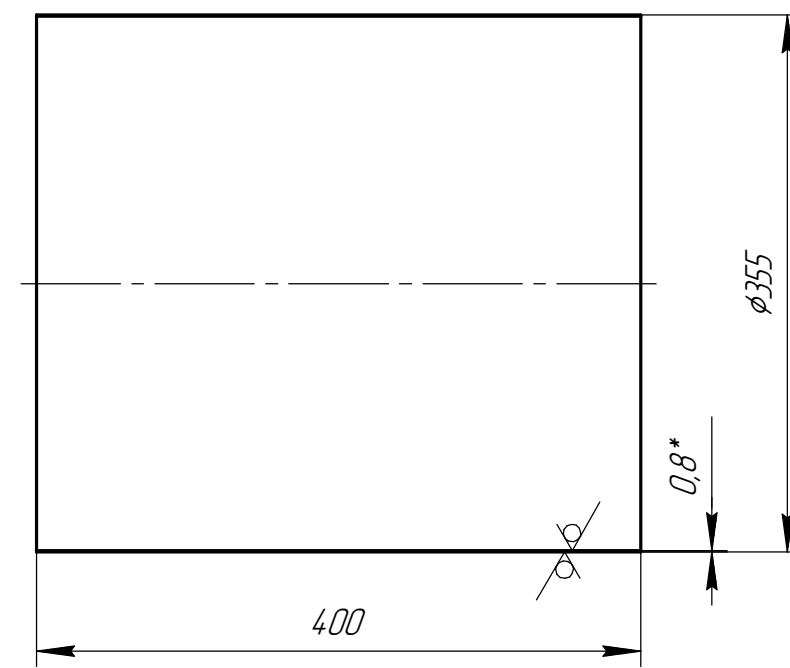
Дет. поз. 9 (1:5)
