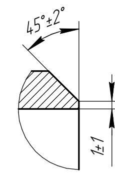
A(2:1)
